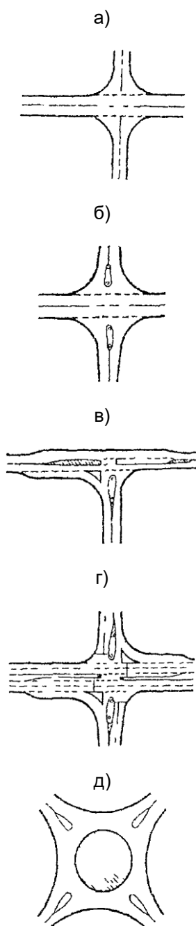
Рис. 8.2. Схемы планировочных решений пересечений: а - простое необорудованное пересечение; б - частично канализированное пересечение с направляющими островками
