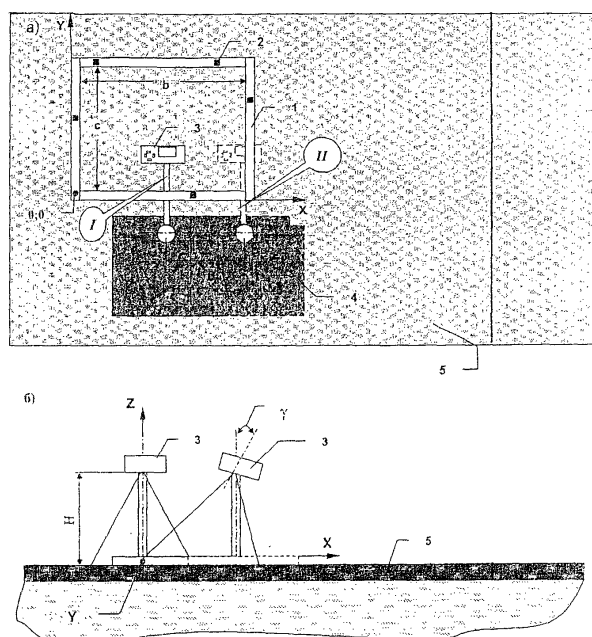
Рис. П-7.1. Схема элементов фотосъемки:
