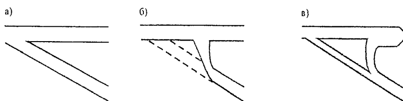
Рис. 8.4. Способы реконструкции примыканий дорог: а - неправильная планировка примыкания; б - улучшение условий движения путем смещения места примыкания; в - устройство дополнительной полосы
