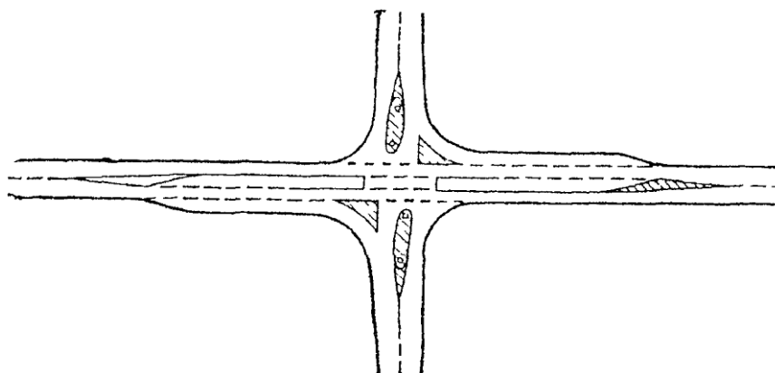
Рис. 8.13. Выделение островков на проезжей части разметкой
