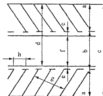
Рис. 11.7. Схемы расстановки автомобилей на стоянках: а - прямоугольная; б - косоугольная
