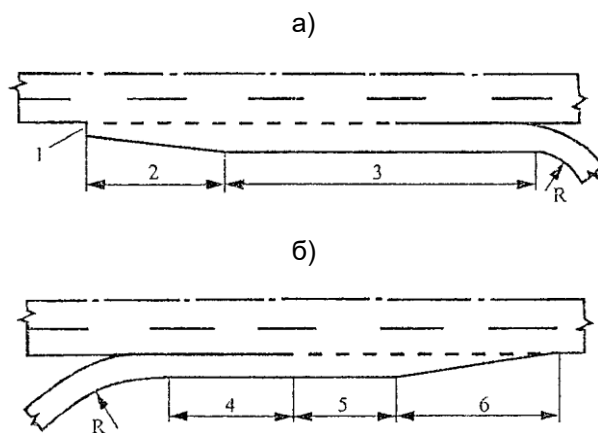
Рис. 9.1. Элементы полос торможения (а) и разгона (б): 1 - уступ шириной 0,5 м; 2 - участок смены полосы движения (отгон ширины полосы); 3 - участок снижения скорости; 4 - участок ускорения; 5 - участок маневрирования
