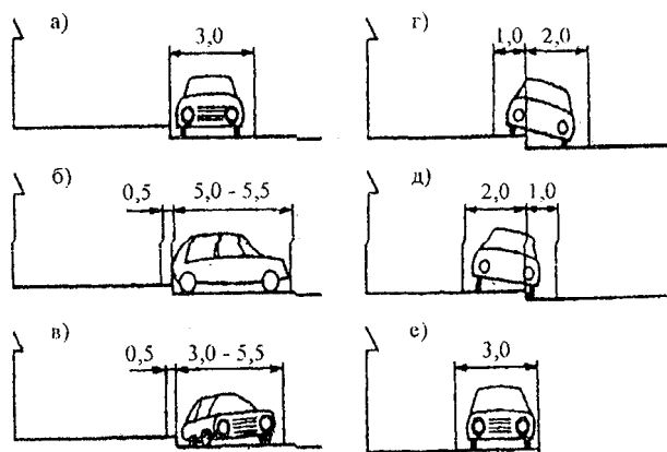
Рис. 11.6. Размещение стоянок в пределах улиц: а - расстановка автомобилей вдоль улиц; б - поперечная расстановка; в - расстановка под углом; г - д - частичное использование тротуара; е - расстановка на тротуаре
