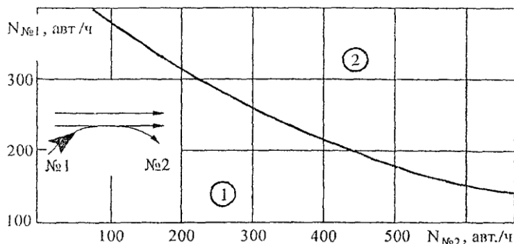
Рис. 9.3. Диаграмма применимости различных типов левоповоротных съездов: 1 - левоповоротный съезд пересечения "клеверный лист"; 2 - полупрямой левоповоротный съезд; N_{№1} , N_{№2} - интенсивности движения по съездам N 1 и N 2
