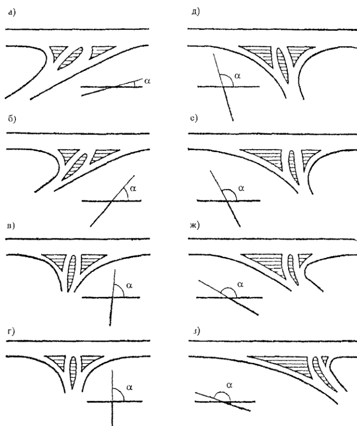
Рис. 8.12. Изменение планировки в зависимости от угла пересечения дорог: а - \alpha = 30^\circ ; б - \alpha = 30-45^\circ ; в - \alpha = 50-75^\circ ; г - \alpha = 90^\circ ; д - \alpha = 115^\circ ; е - \alpha = 135^\circ ; ж - \alpha = 150^\circ ; з - \alpha > 150^\circ
