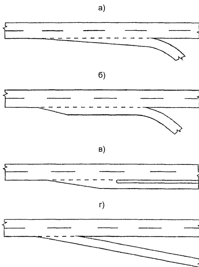
Рис. 9.2. Типы переходно-скоростных полос
