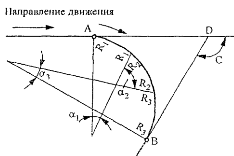
Рис. 8.3. Схема для расчета коробовой кривой
