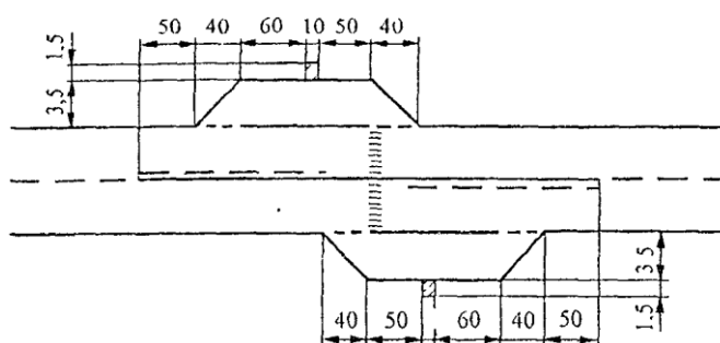
Рис. 11.9. Планировка автобусных остановок в населенных пунктах
