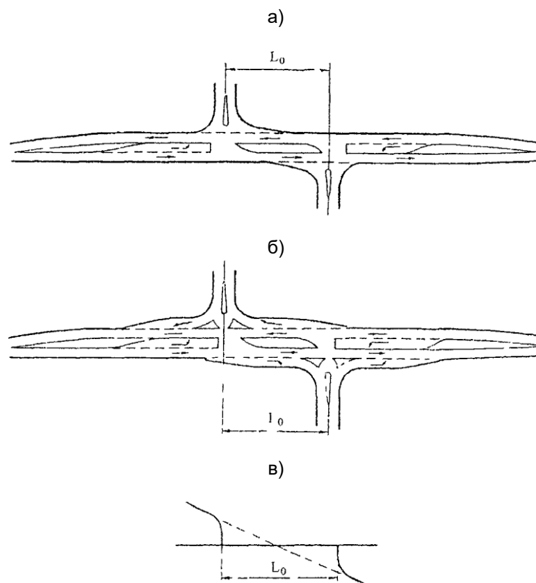
Рис. 8.6. Перестройка пересечения на два смещенных примыкания: а - без переходно-скоростных полос; б - с переходно-скоростными полосами; в - схема изменения пересечения
