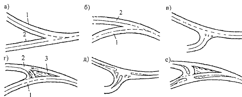
Рис. 8.5. Рекомендуемые схемы планировки пересечений в одном уровне на обходе населенных пунктов: а, б - неправильная схема без разделения дорог на главную и второстепенную; в, г - рекомендуемые схемы при невысокой интенсивности движения на второстепенной дороге; д, е - то же, при высокой интенсивности; 1 - главная дорога; 2 - второстепенная дорога; 3 - распределительная полоса
