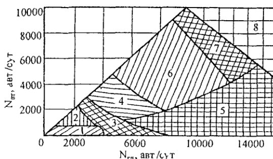
Рис. 8.1. Номограмма для выбора типа планировочных решений пересечений:
