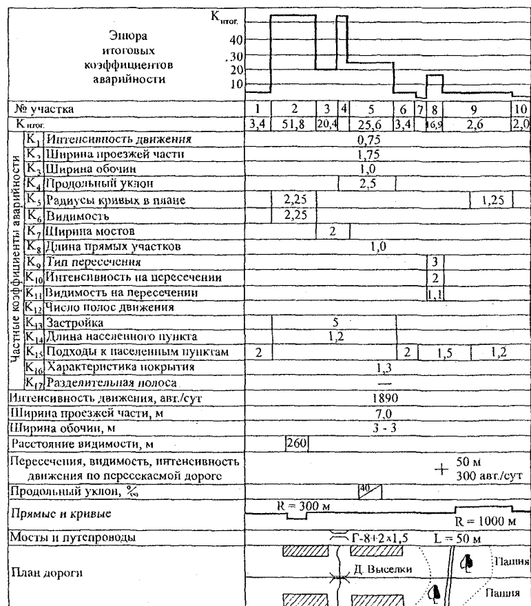
Рис. 1.2. Пример графика итогового коэффициента аварийности
