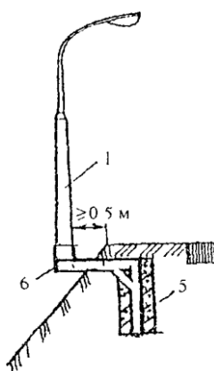
Рис. 15.1. Схема заделки в грунт опор освещения: а - при благоприятных условиях; б - в пучинистых грунтах; в - при наличии подземных коммуникаций; 1 - опора; 2 - оголовок; 3 - свая; 4 - деревянный короб; 5 - бетонный фундамент; 6 - металлический Г-образный фундамент
