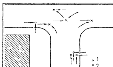
Рис. 8.9. План пересечения с нанесенными на него схемами дорожно-транспортных происшествий:
