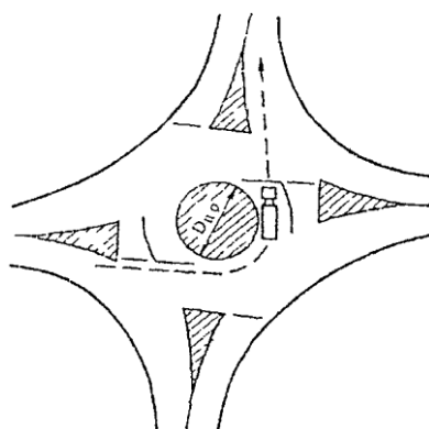
Рис. 8.17. Схема расположения автопоезда в зоне
