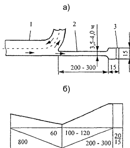
Рис. 5.1. Схема аварийного съезда: а - план; б - продольный профиль; 1 - основная дорога; 2 - аварийный съезд; 3 - песчаный вал
