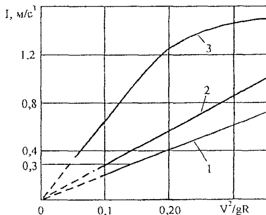
Рис. 4.2. График для определения расчетного нарастания центробежного ускорения
