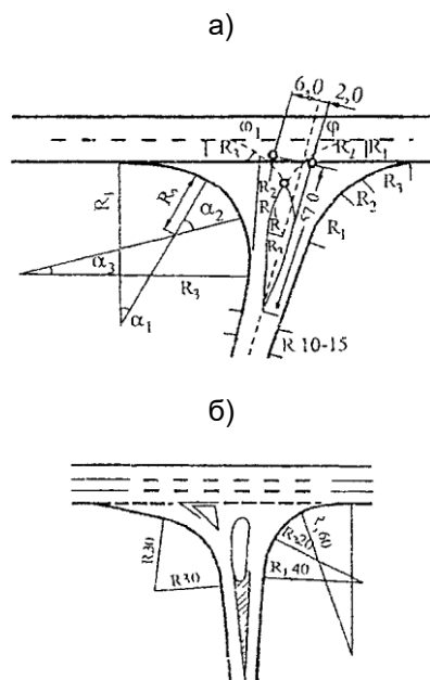
Рис. 8.10. Расположение островков на второстепенной дороге:
