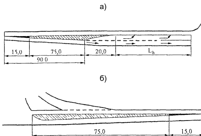
Рис. 8.11. Расположение островков на главной дороге: а - левоповоротный островок; б - направляющий островок
