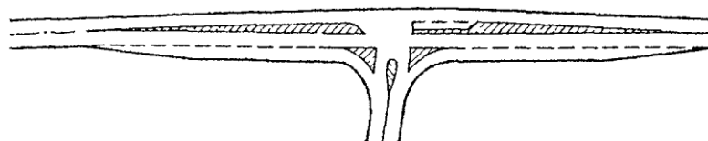
Рис. 8.8. Направляющие островки на примыкании в одном уровне
