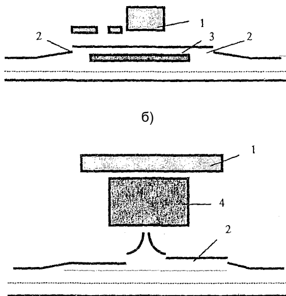
Рис. 11.3. Схемы расположения автомобильных стоянок в населенных пунктах: а - стоянка линейного типа; б - площадка для стоянки автомобилей; 1 - объекты обслуживания; 2 - переходно-скоростные полосы; 3 - разделительные полосы; 4 - площадка для стоянки автомобилей
