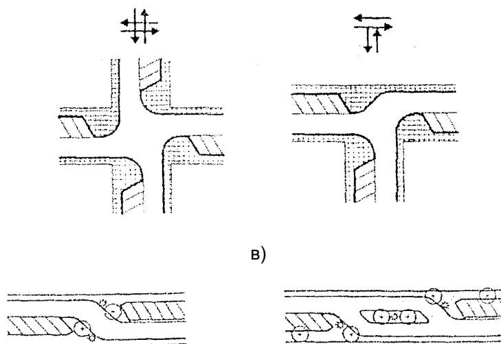
Рис. 11.10. Мероприятия по "успокоению движения" на участках дорог: а - изменение геометрии проезжей части (черным обозначена зона движения, белым - зона парковки), озеленение или другие элементы благоустройства; б - варианты изменения конфигурации пересечения и примыкания с размещением мест для парковки и зон пешеходного движения; в - варианты излома плана проезжей части с размещением мест для парковки
