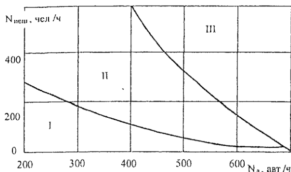
Рис. 11.2. Области применения пешеходных переходов различных типов: I - нерегулируемые переходы; II - светофорное регулирование; III - внеуличные пешеходные переходы
