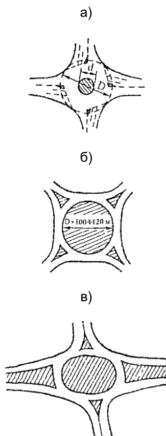
Рис. 8.14. Планировочные схемы кольцевых пересечений: а - с малым островком; б - с большим островком; в - с эллиптическим
