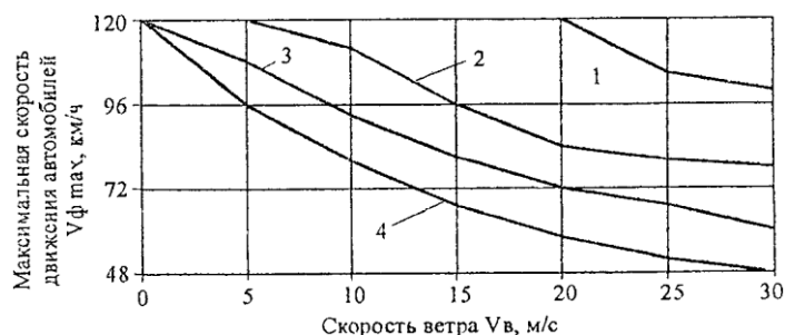
Рис. 1.3. Зависимости максимальной безопасной скорости движения автомобилей от скорости ветра: 1, 3 - для легковых автомобилей с передним расположением двигателя, время реакции водителя 1,0 и 1,5 с соответственно; 2, 4 - то же, для автомобилей с задним расположением двигателя
