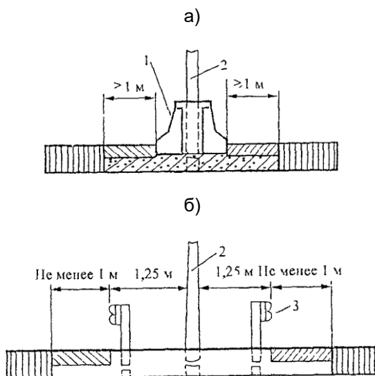
Рис. 15.2. Схема установки опор освещения и ограждений на разделительной полосе: 1 - железобетонный блок; 2 - опора; 3 - барьерное металлическое ограждение
