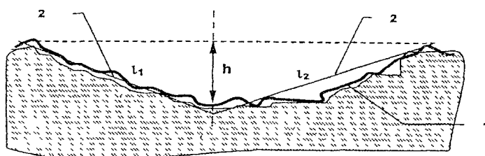
Рис. П-7.2. Схема к расположению опорной рамки для оценки колеи: 1 - профиль колеи; 2 - линии осредненного поперечного уклона колеи; h - глубина колеи; l - уклон
